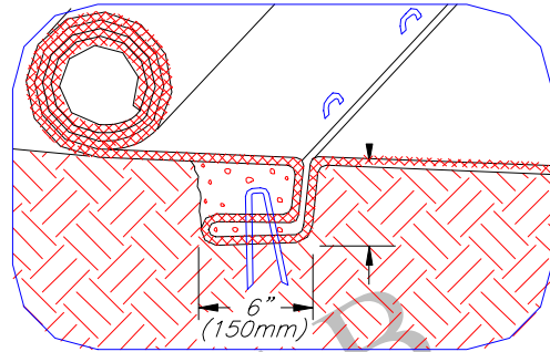
Förankring av tvärskarvar
