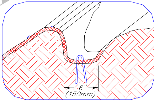
Längsgående förankring vid krön
